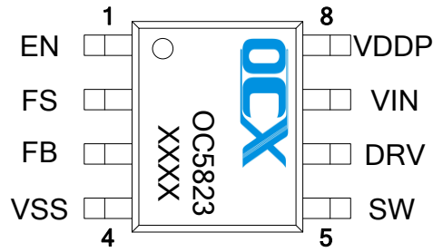
SOP8
